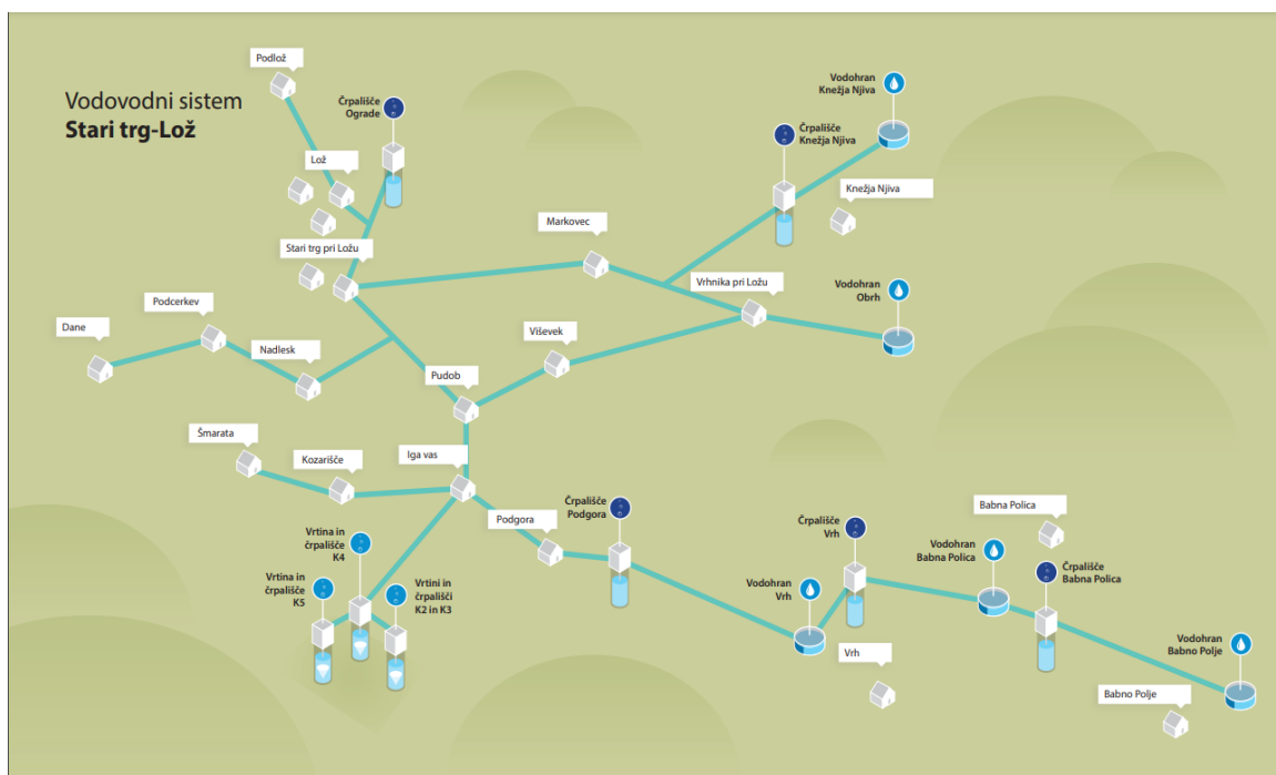
Slika 1: Vodovodni sistem Stari trg-Lož, ki ga upravlja JP Komunala Cerknica
