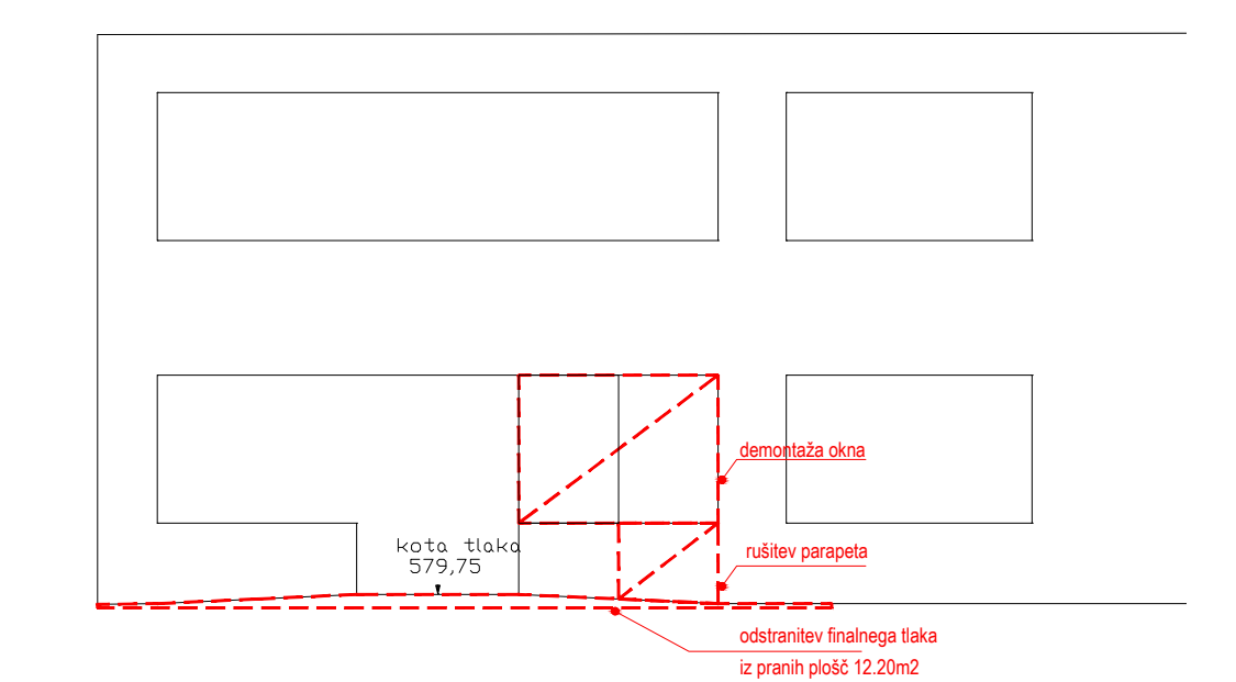
Fasada obstoječega objekta - odstranitvena dela m=1:100
