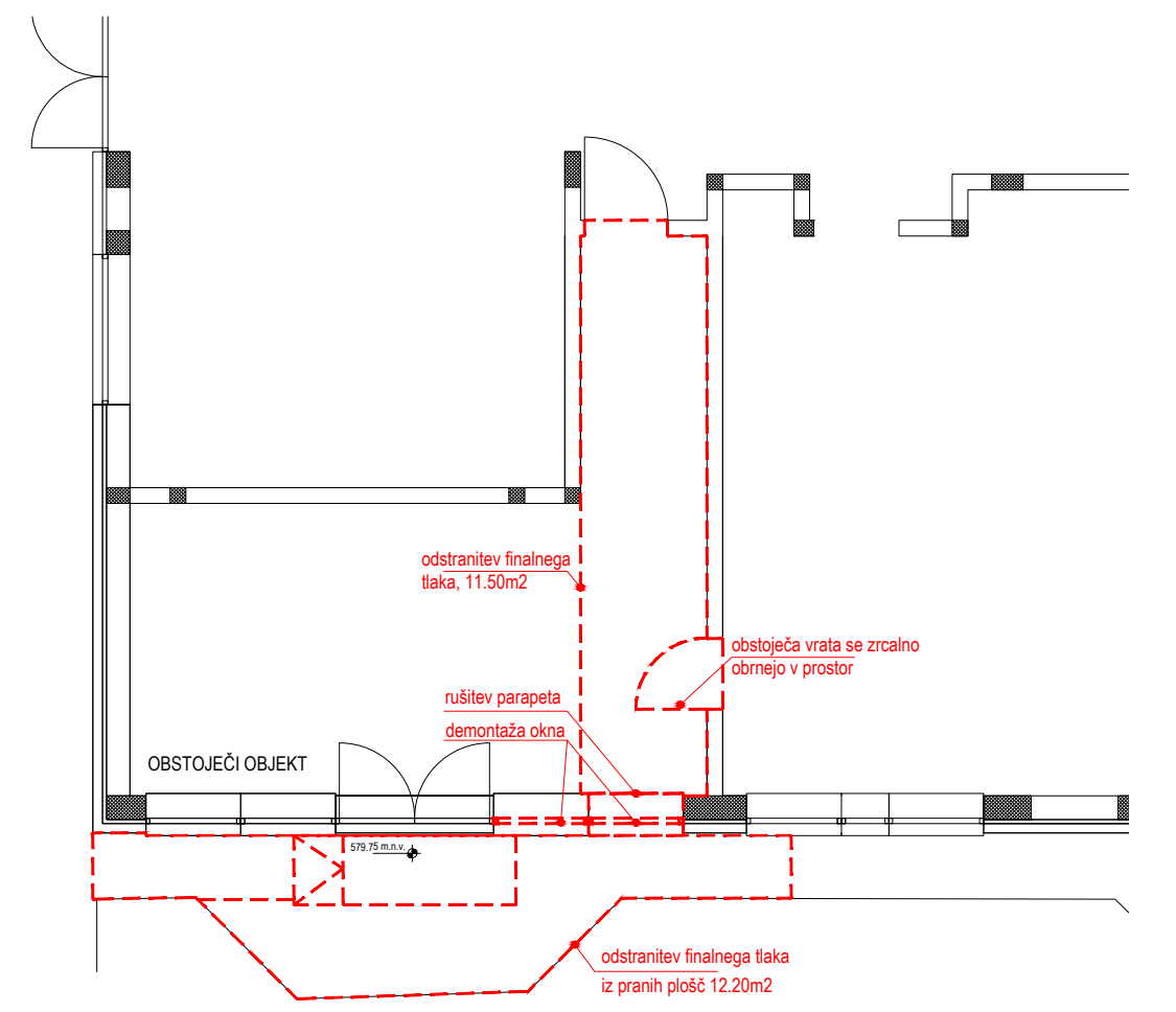
Tloris obstoječega objekta - odstranitvena dela m=1:100
